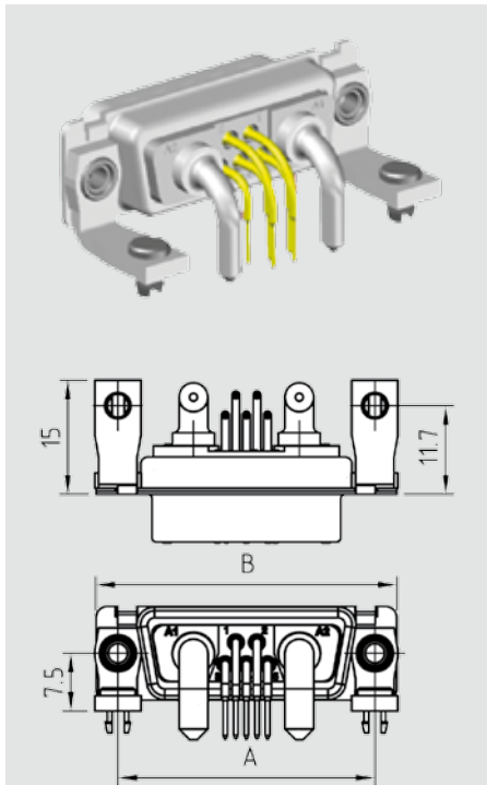
Polanordnung Arrangement
